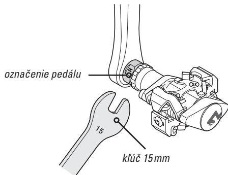
obrázok 29 - montáž pedálu
